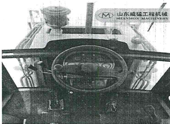
INVERSOR DE MARCHA FRENTE E RÉ AÇIONADO POR ALAVANCA NA COLUNA DE DIREÇÃO
